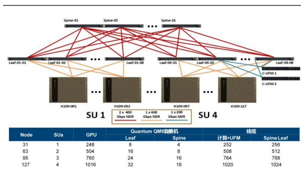
图 13: 英伟达 H100 4SU 方案示意图
