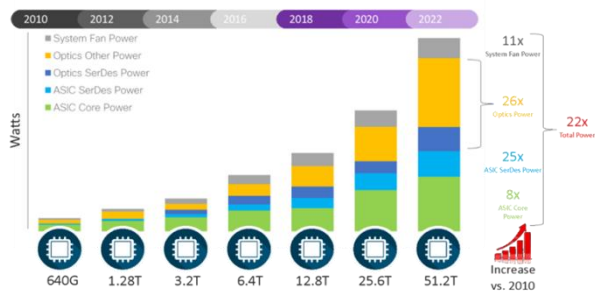
图 15: SerDes 速率提升下功耗持续提升
