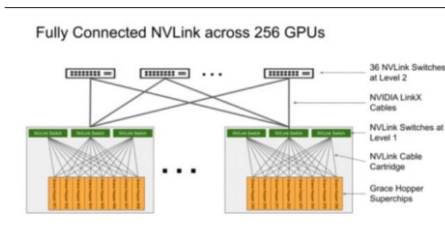
图 14: 英伟达 GH200 示意图
