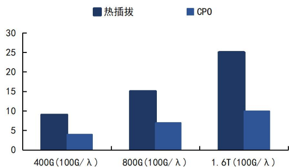
图 19: CPO 能显著降低光模块功耗
