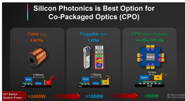
图 18: 硅光是 CPO 的最佳选择
