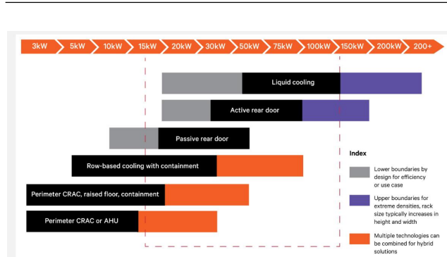
图24：单机柜功率密度与冷却方式演变
