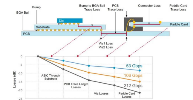
图 16: erDes 速率提升, 电 I/O 接口损耗加大
